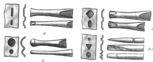
3 сурет – Шекігіштер түрлері және металл бетіне салынатын іздер: а – жұмсалғыш; ә – лошатник; б – пурошник; в – конфарник- г – сотан
